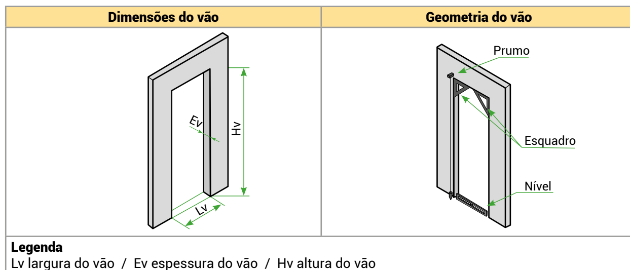
Figura 2 - Vão da porta
