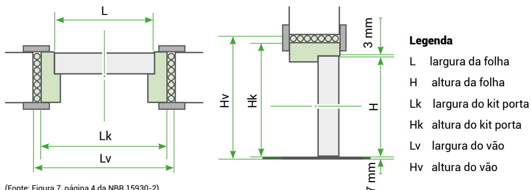
Figura 1 – Dimensões do kit porta de giro com 1 folha
